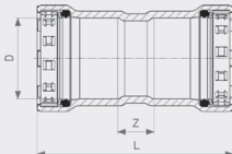
Megapress supistusmuhvi - seostamatonta terästä, sinkki-nikkeli-päällyste malli 4215.7
