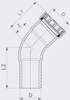
Megapress käyrä 45° - seostamatonta terästä, sinkki-nikkeli-päällyste malli 4226.1
