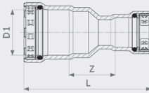
Megapress supistusmuhvi - seostamatonta terästä, sinkki-nikkeli-päällyste malli 4215.2
