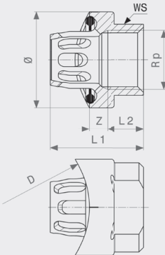
Megapress pistoliitin - seostamaton terästä, sinkki-nikkeli-päällyste malli 4212.2
