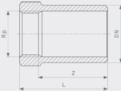
Megapress pistoliitin - seostamaton terästä, sinkki-nikkeli-päällyste malli 4212.5
