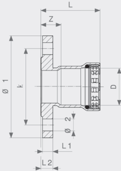
Megapress laippaliitin - seostamaton terästä, sinkki-nikkeli-päällyste malli 4259.1
