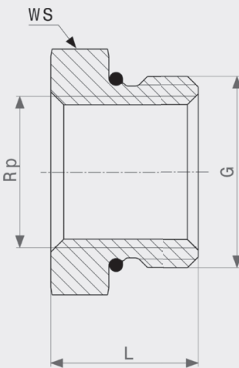
Supistus - punametallia malli 3241.1
