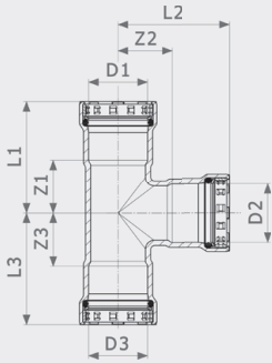
Megapress T-yhde - seostamaton terästä, sinkki-nikkeli-päällyste malli 4218
