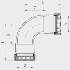
Megapress käyrä 90° - seostamatonta terästä, sinkki-nikkeli-päällyste malli 4216
