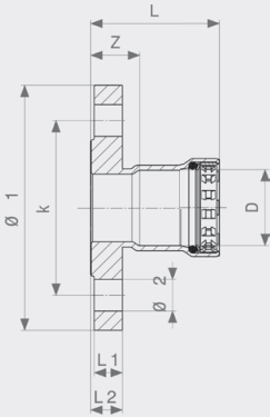
Megapress laippaliitin - seostamaton terästä, sinkki-nikkeli-päällyste malli 4259
