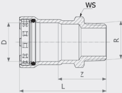
Megapress nippa - seostamatonta terästä, sinkki-nikkeli-päällyste malli 4211
