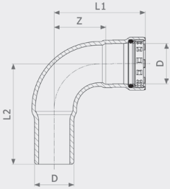
Megapress käyrä 90° - seostamatonta terästä, sinkki-nikkeli-päällyste malli 4216.1
