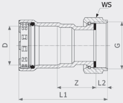
Megapress yhdistäjä - seostamaton terästä, sinkki-nikkeli-päällyste malli 4263
