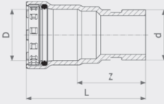
Megapress nippa - seostamaton terästä, sinkki-nikkeli-päällyste malli 4213.1
