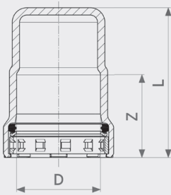
Megapress hattu - seostamaton terästä, sinkki-nikkeli-päällyste malli 4256
