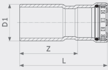
Megapress supistus - seostamatonta terästä, sinkki-nikkeli-päällyste malli 4215.1
