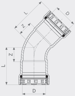
Megapress käyrä 45° - seostamatonta terästä, sinkki-nikkeli-päällyste malli 4226
