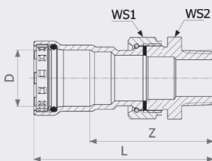
Megapress yhdistäjä - seostamatonta terästä, sinkki-nikkeli-päällyste malli 4265
