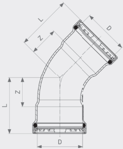
Megapress S XL käyrä 45° - seostamatonta terästä, sinkki-nikkeli-päällyste malli 4226XL
