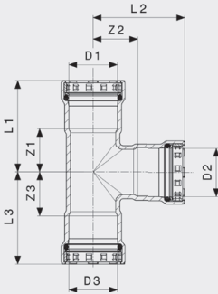
Megapress S T-yhde - seostamaton terästä, sinkki-nikkeli-päällyste malli 4318
