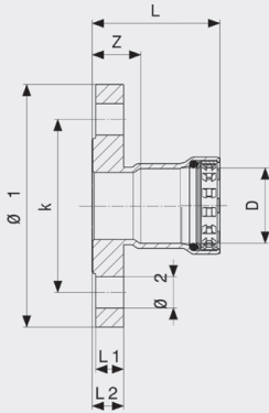
Megapress S laippaliitin - seostamaton terästä, sinkki-nikkeli-päällyste malli 4359.6
