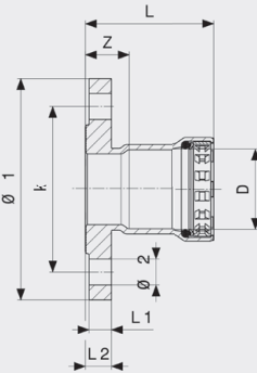
Megapress S laippaliitin - seostamatonta terästä, sinkki-nikkeli-päällyste malli 4359.1
