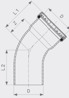
Megapress S XL käyrä 45° - seostamaton terästä, sinkki-nikkeli-päällyste malli 4226.1XL
