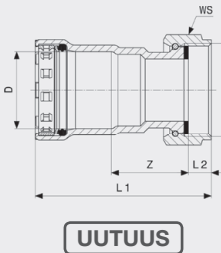
Megapress S yhdistäjä - seostamatonta terästä, sinkki-nikkeli-päällyste malli 4363
