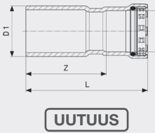
Megapress S supistus - seostamatonta terästä, sinkki-nikkeli-päällyste malli 4315.1
