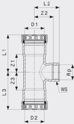
Megapress S T-yhde - seostamaton terästä, sinkki-nikkeli-päällyste malli 4317.2
