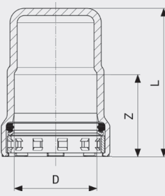
Megapress S hattu - seostamatonta terästä, sinkki-nikkeli-päällyste malli 4356
