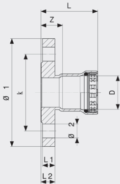
Megapress S laippaliitin - seostamatonta terästä, sinkki-nikkeli-päällyste malli 4359
