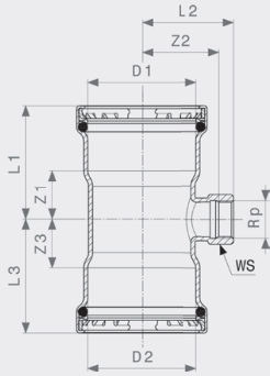
Megapress S XL T-yhde - seostamaton terästä, sinkki-nikkeli-päällyste malli 4217.2XL
