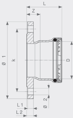
Megapress S XL laippaliitin - seostamatonta terästä, sinkki-nikkeli-päällyste malli 4259.1XL
