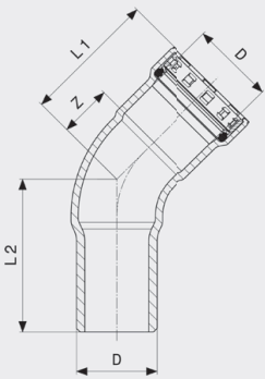
Megapress S käyrä 45° - seostamatonta terästä, sinkki-nikkeli-päällyste malli 4326.1
