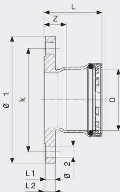
Megapress S XL laippaliitin - seostamaton terästä, sinkki-nikkeli-päällyste malli 4259.6XL
