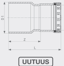
Megapress S XL supistus - seostamatonta terästä, sinkki-nikkeli-päällyste malli 4215.1XL
