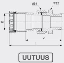
Megapress S yhdistäjä - seostamatonta terästä, sinkki-nikkeli-päällyste malli 4365
